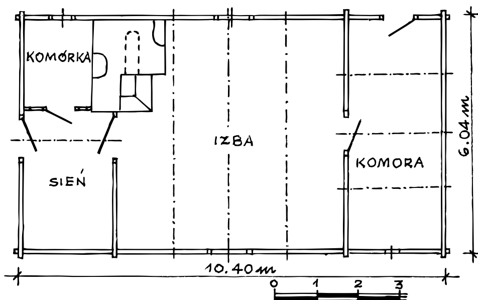
Ryc. 2. Radkowiec nr 86, gm. Chęciny. Dom z 1881 r. Rzut przyziemia. Stan w 1975 r. Rys. B. Szurowa, X 1975 r. Odrys E. Traczyński.
