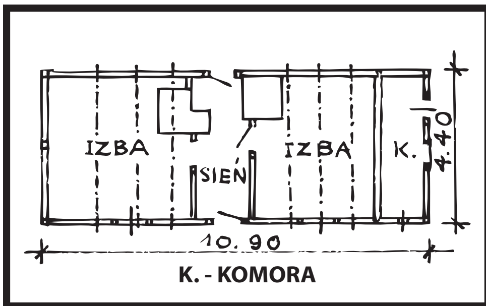
Ryc. 4. Chęciny, ul. Strażacka nr 3. Dom prawdopodobnie z I poł. XIX w. Rzut przyziemia. Stan w 1983 r. Odrys E. Traczyński.
