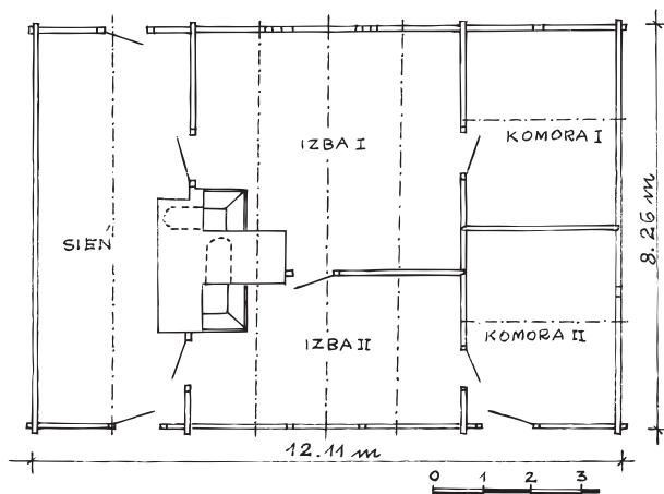
Ryc. 13. Radkowie nr 21, gm. Chęciny. Dom z 1879 r. Rzut przyziemia. Stan w 1975 r. Rys. B. Szurawa, X 1975 r. Odrys E. Traczyński.
