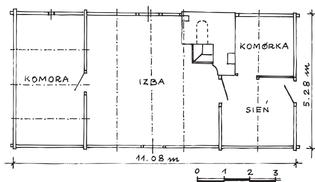
Ryc. 11. Radkowice nr 70, gm. Chęciny. Dom z 1876 r. Rzut przyziemia. Stan w 1975 r. Rys. B. Szurowa, X 1975 r. Odrys E. Traczyński.
