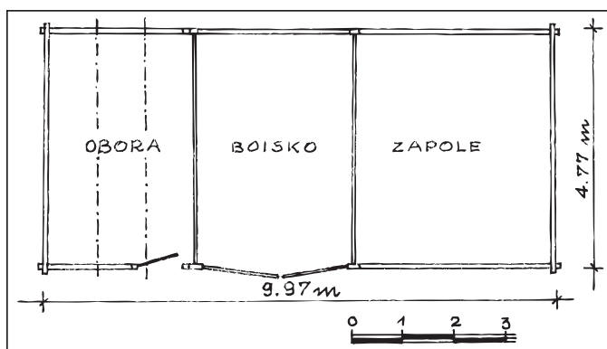
Ryc. 7. Radkowice nr 14, Gm. Chęciny. Opora ze stodołą z II połowy XIX w. Stan w 1975 r.
